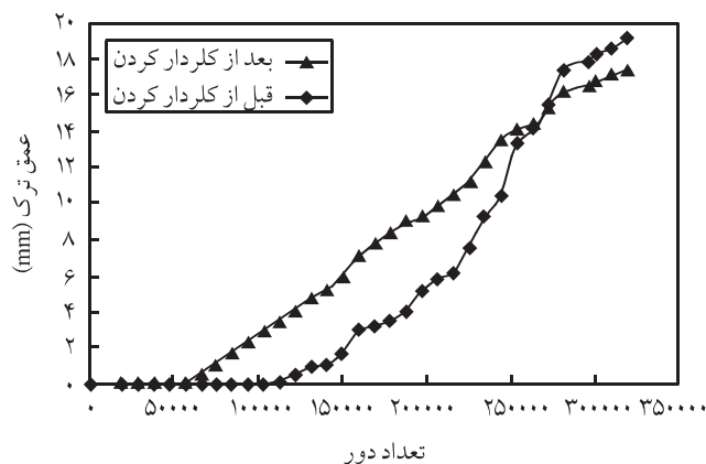
شکل ۹ تغییرات خستگی آمیزه NR/CR پس از کلردار کردن.
