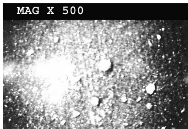
شکل ۲ تصویر SEM سطح نمونه NR/CR پس از ۵ min کلردار کردن با بزرگنمایی ۵۰۰.
