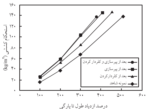
شکل ۸ تغییر خواص کششی پس از کلردار کردن در آمیزه NR/CR
