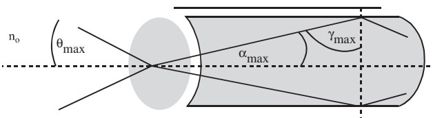
شکل ۴- نمودار زاویه پذیرش و گشودگی عددی [۱].
