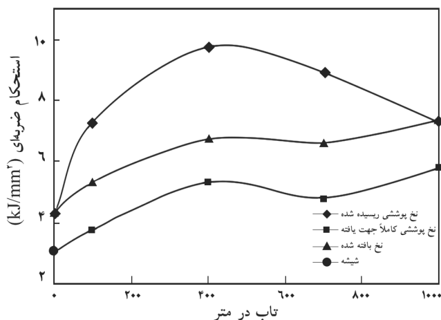
شکل ۷- استحکام ضربه‌ای قطعات کامپوزیتی تقویت شده با انواع نخهای پوششی در تابهای مختلف و مقایسه آنها با قطعه کامپوزیتی تقویت شده با الیاف شیشه.
