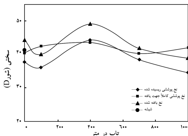
شکل ۸- سختی قطعات کامپوزیتی تقویت شده با انواع نخهای پوششی در تابهای مختلف و مقایسه آنها با قطعه کامپوزیتی تقویت شده با الیاف شیشه.
