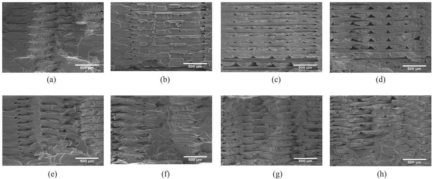
شکل ۷- تصاویر SEM از سطح شکست تمام نمونه‌های چاپ‌شده در زاویه‌های رشته‌نشانی 0/90^\circ (بالا) و 45/-45^\circ (پایین) با ضخامت لایه 0.1 \text{ mm} دارای مقادیر مختلف نانوذرات پس از آزمون کشش: (a)، (e) 0 \text{ wt}\% ، (b)، (f) 1 \text{ wt}\% ، (c)، (g) 3 \text{ wt}\% ، و (d)، (h) 5 \text{ wt}\% .
