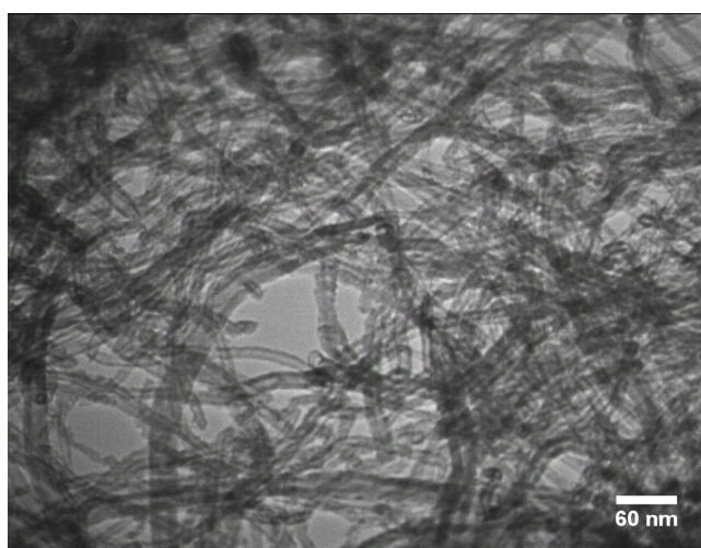
شکل ۲- تصویر TEM از نانوکامپوزیت دارای ۳٪ وزنی MWCNTs. Fig. 2. TEM image of the nanocomposite containing 3 wt% MWCNTs.
