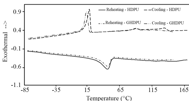
شکل ۴- دمانگاشت های مراحل گرمایش مجدد و سرمایش آزمون DSC برای نمونه های HDPU و GHDPU.
