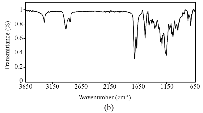
شکل ۱- طیف‌های FTIR نمونه‌ها: (a) TDPU و (b) HDPU.
