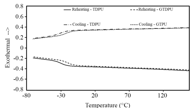
شکل ۳- دمانگاشت های مراحل گرمایش مجدد و سرمایش آزمون DSC برای نمونه های TDPU و GTDPU.
