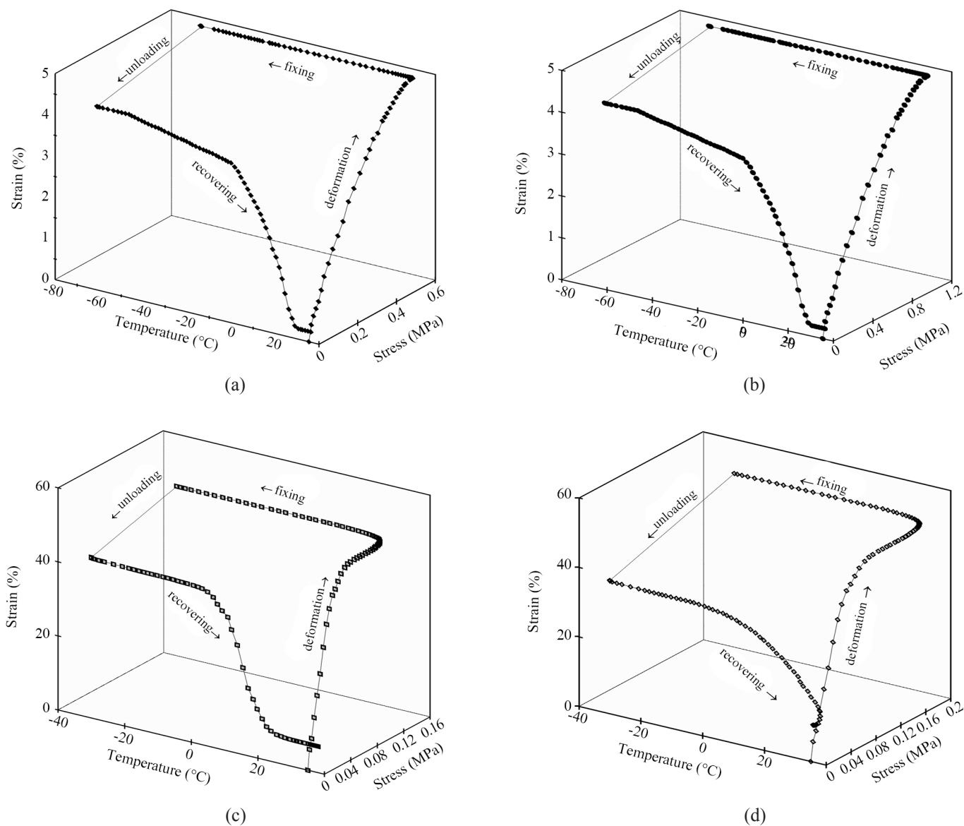
شکل ۶- منحنی‌های دما-تنش-کرنش نمونه‌های حافظه شکلی: (a) HDPU، (b) GHDPUs، (c) TDPU و (d) GTDPU.
