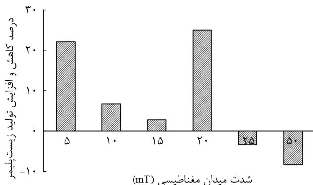
شکل ۲- درصد افزایش و کاهش مقدار زیست‌پلیمر در میدان‌های مغناطیسی مختلف در مقایسه با نمونه شاهد.
